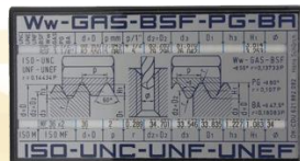
TP-2(ねじ山公差表)
